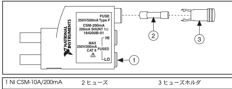
図7 ヒューズを取り外す
