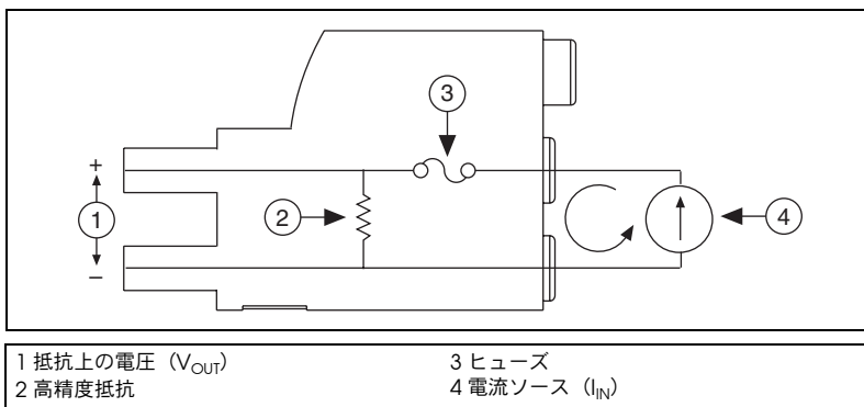
図 5 CSM 内部構造
