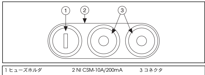
図 6 CSM ヒューズホルダの位置 (前面図)
