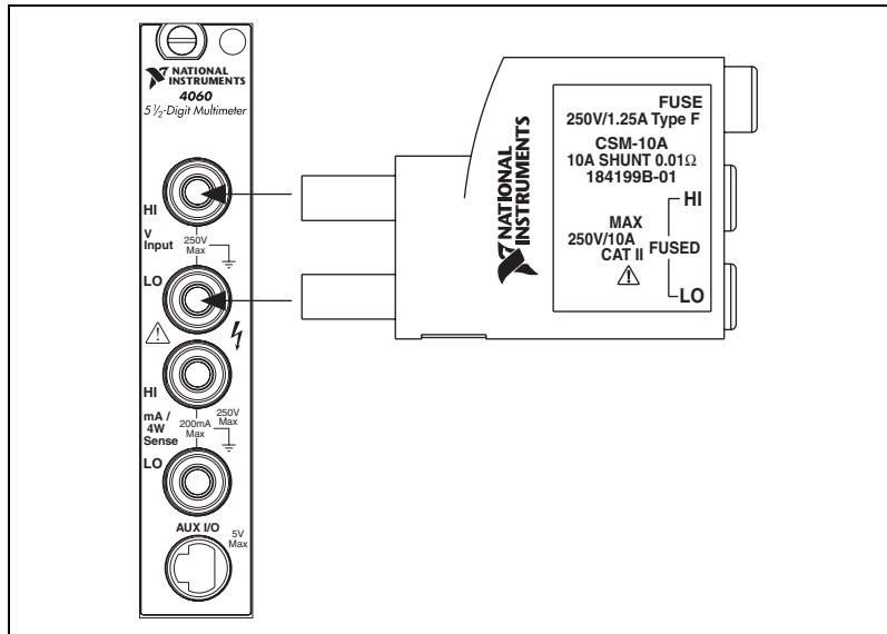
図 2 CSM を NI 4060 に接続する
