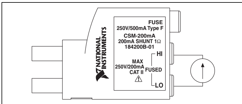
図 4 電流を CSM に接続する
