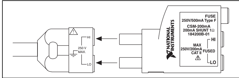
図 1 CSM を NI 4050 付属の P4-BJ2 ケーブルに接続する
