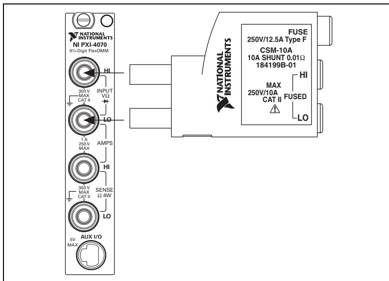
図 3 CSM を NI 4070 に接続する
