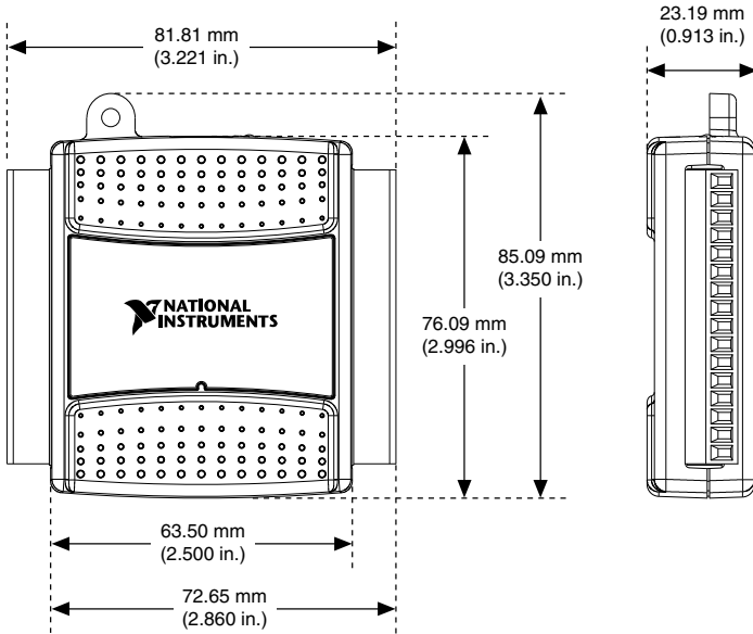
図 1. USB-6009 外形寸法
