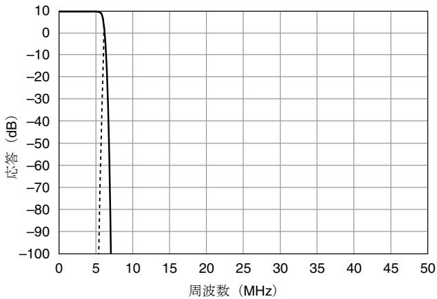
図 7 DDC フィルタ性能、10 MHz スパン
