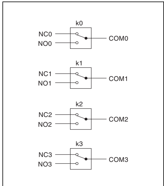
図 4 NI PXI-2548 電源投入時の状態
