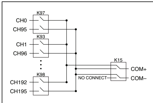
図 1 NI PXI-2575 電源投入時の状態
