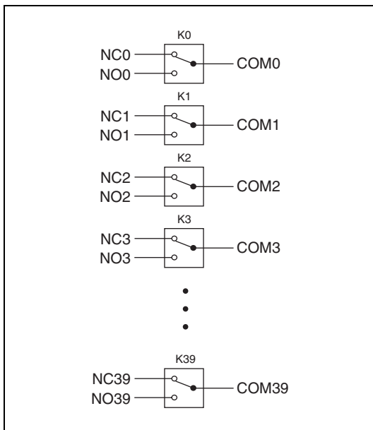
図 1 NI PXI-2570 電源投入時の状態
