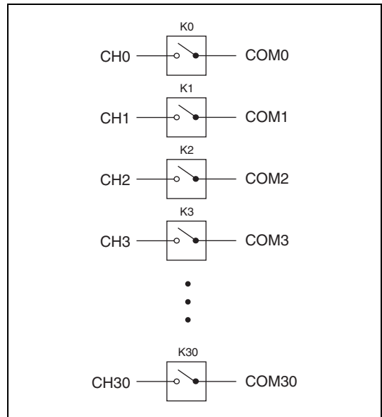
図 1 NI PXI-2568 電源投入時の状態
