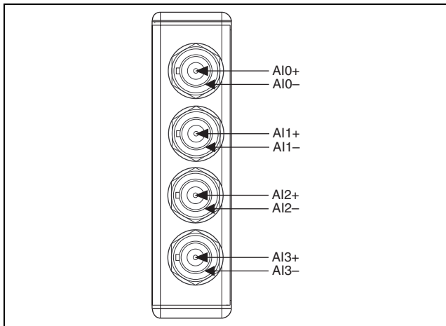
그림 1. NI 9233 커넥터 할당
