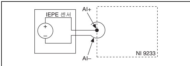
그림 3. 플로팅 IEPE 센서를 NI 9233 에 연결하기
