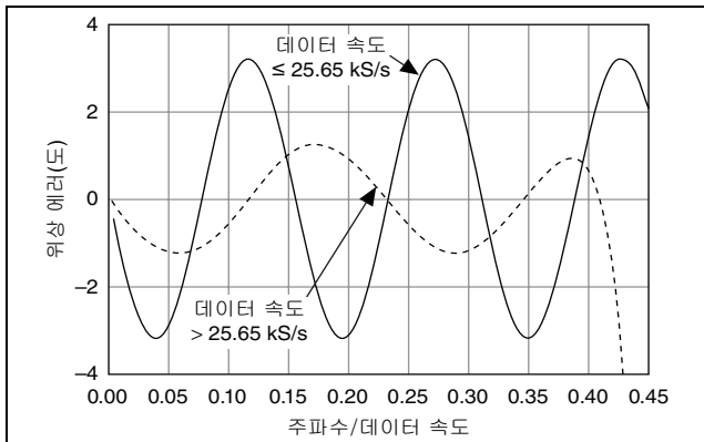
그림 6. NI 9233의 위상 비선형도
