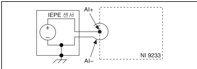
그림 2. 접지된 IEPE 센서를 NI 9233 에 연결하기
