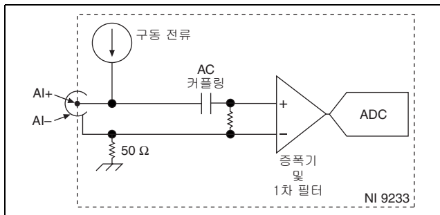
그림 4. NI 9233 의 한 채널에서 입력 회로
