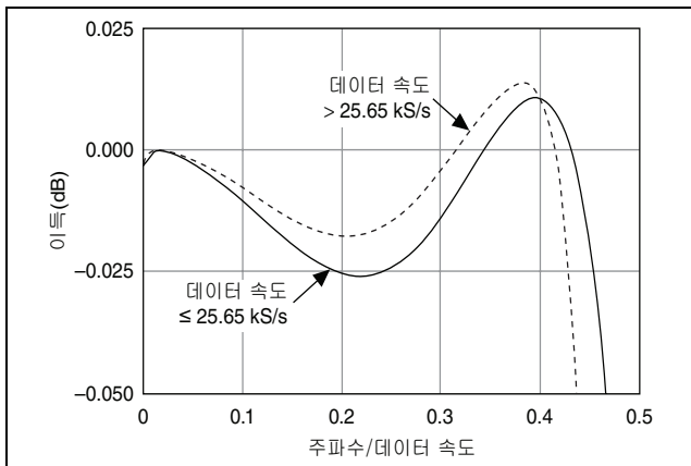
그림 5. NI 9233의 일반적인 통과 대역 평탄도
