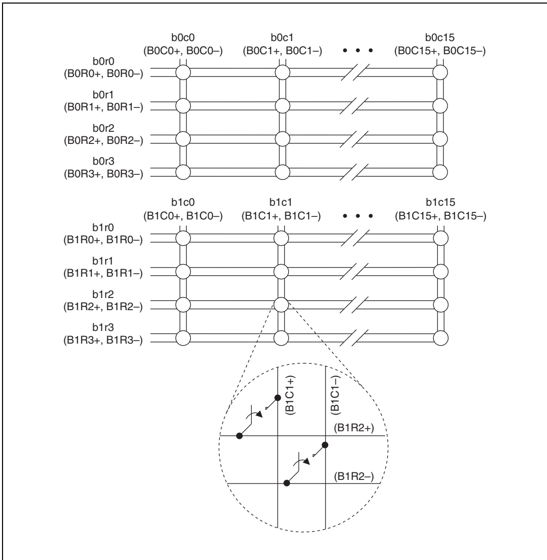
図 1 NI 2529 2 バンク 2 線式 4 × 16 マトリクス構成
