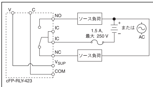
図 2. 基本フィールド接続
