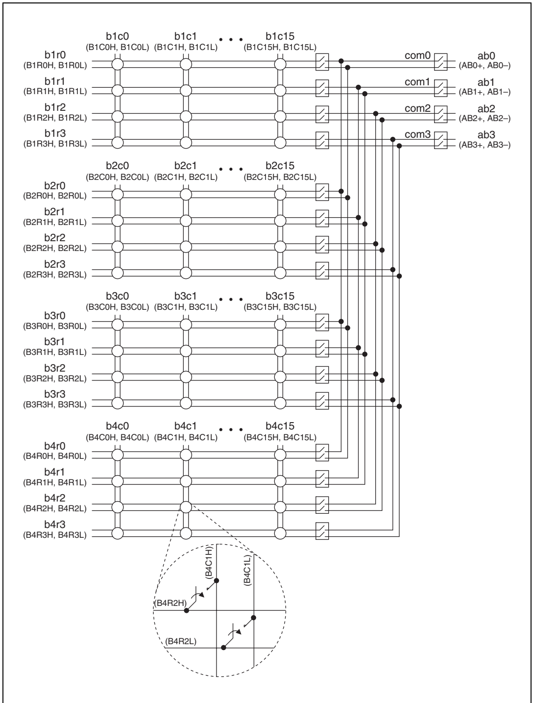
図 1 NI SCXI-1129 4 バンク 2 線式 4 × 16 マトリクストポロジ
