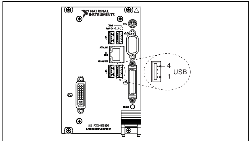
図 3-6 USB コネクタの位置およびピン配列
