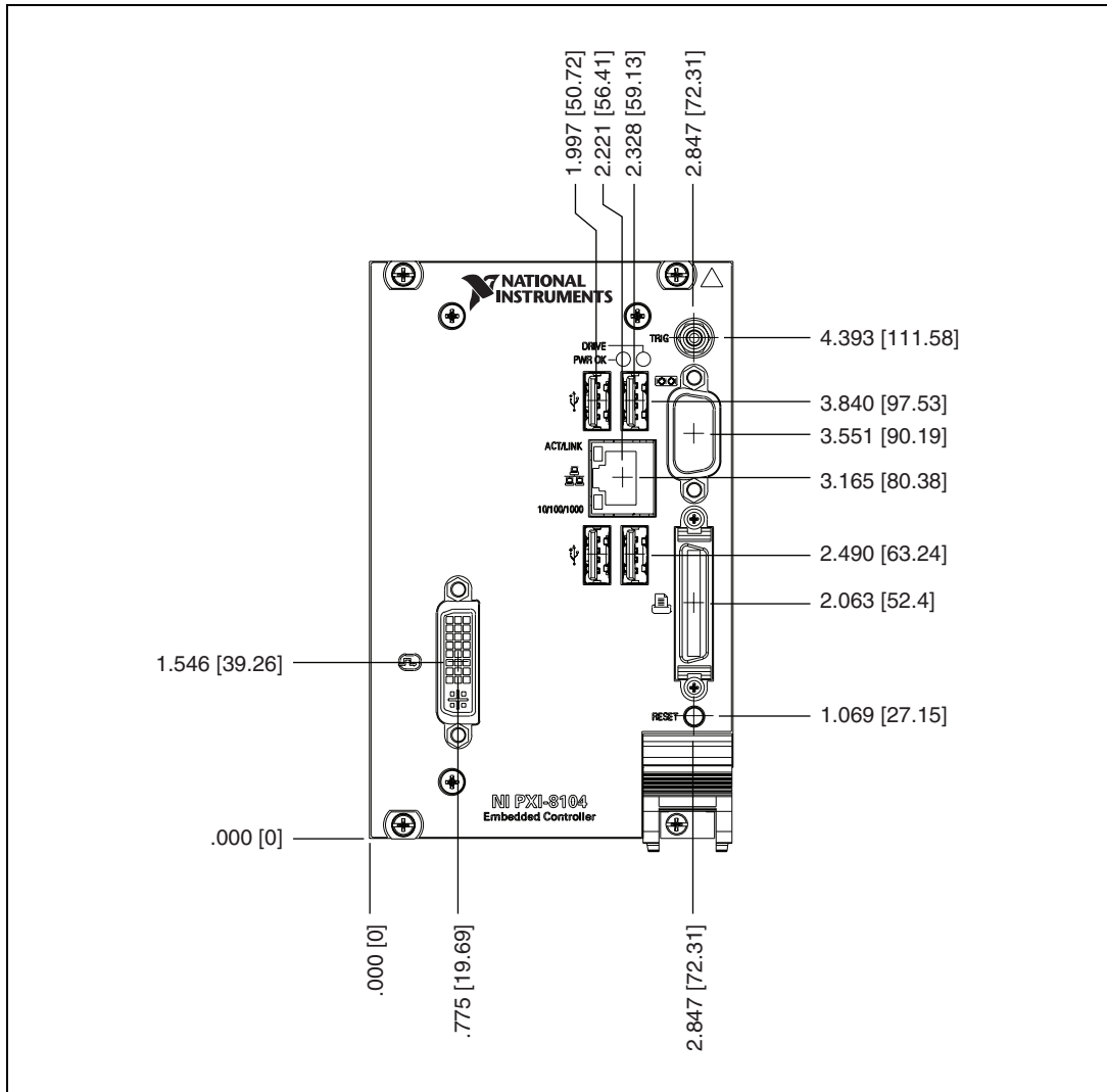
図 3-1 NI PXI-8104 フロントパネルの配置および寸法
