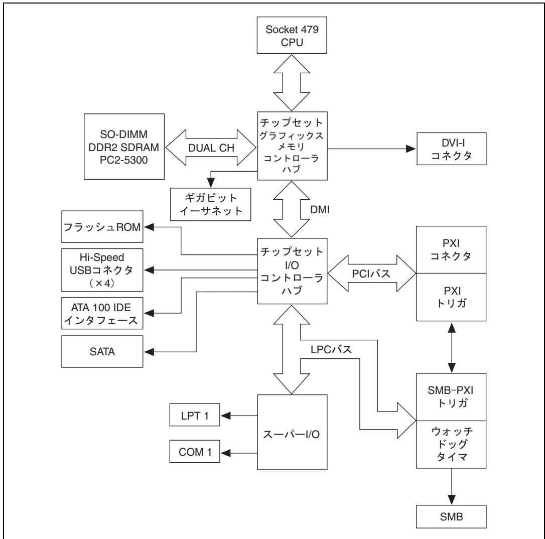
図 1-1 NI PXI-8104 ブロック図
