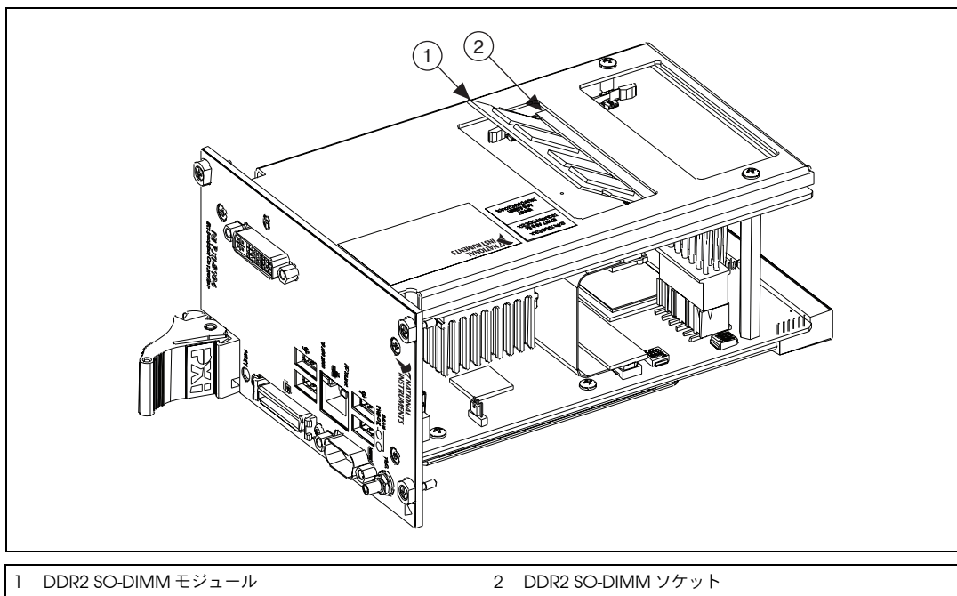
図 2-5 NI PXI-8104 コントローラに DDR2 SO-DIMM を取り付ける
