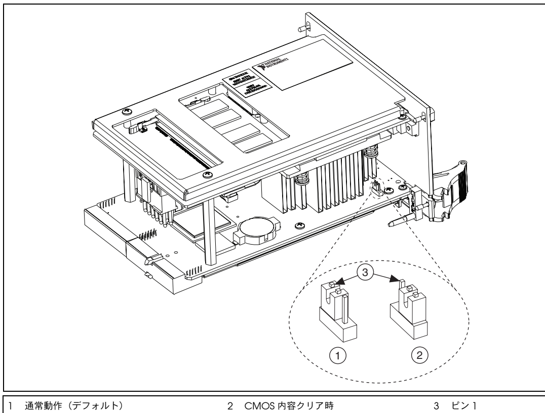
図 2-3 CMOS 内容をクリアする
