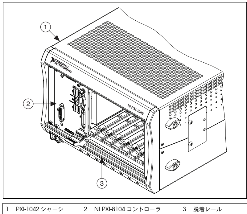
図 2-2 PXI シャーシに取り付けた NI PXI-8104 コントローラ
