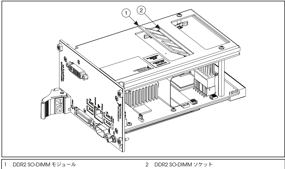
図 4-2 NI PXI-8104 コントローラに DDR2 SO-DIMM を取り付け
