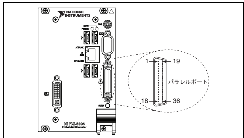
図 3-5 パラレルポートコネクタの位置およびピン配列
