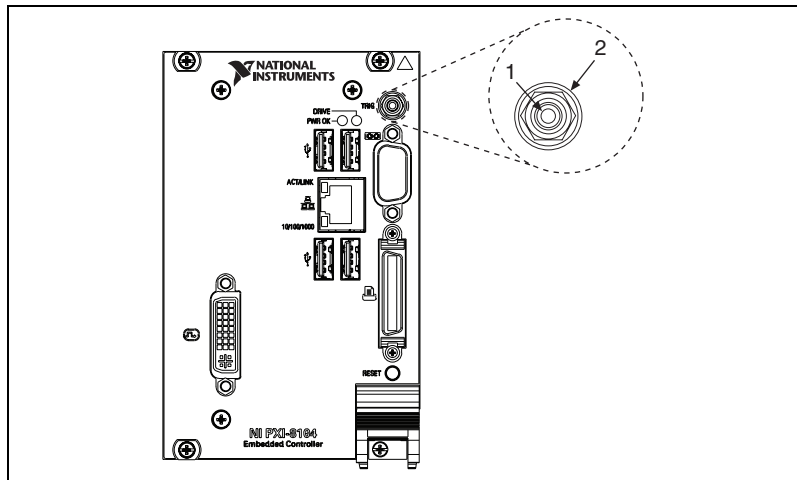
図 3-7 TRG コネクタの位置およびピン配列
