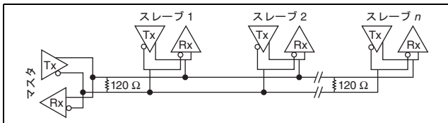
図 5 終端抵抗を使用する 2 線マルチドロップネットワーク
