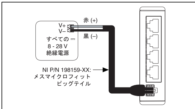
図 2 絶縁電源から NI 9871 に電源を投入する
