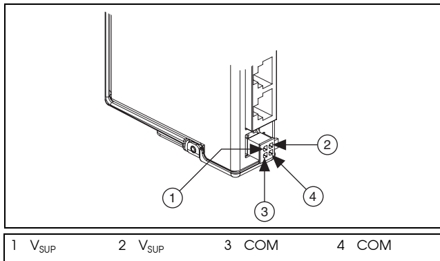
図 1 4 位置外部電源コネクタ
