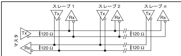
図 4 終端抵抗を使用する 4 線式全二重マルチドロップネットワーク
