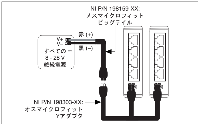
図 3 1つの電源から複数のモジュールに電源を投入する
