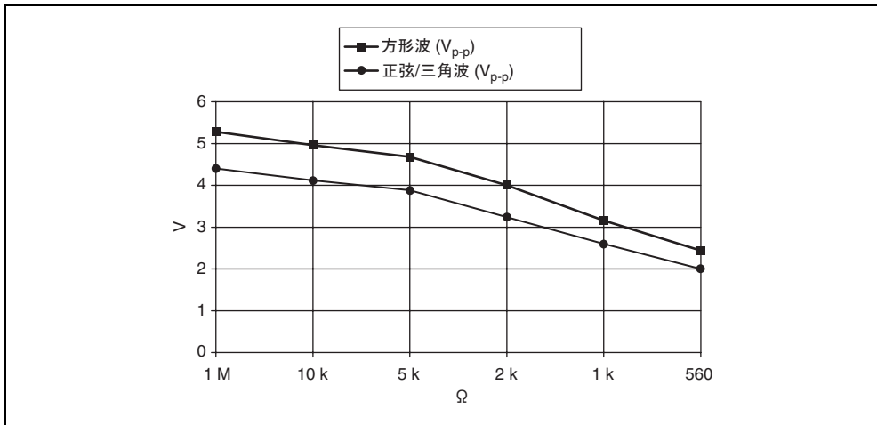
図7 標準最大電圧と負荷インピーダンス
