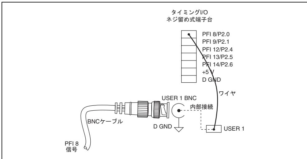
図 6 PFI 8 を USER 1 BNC に接続する
