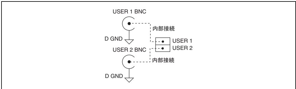
図 5 USER <1..2> BNC 接続
