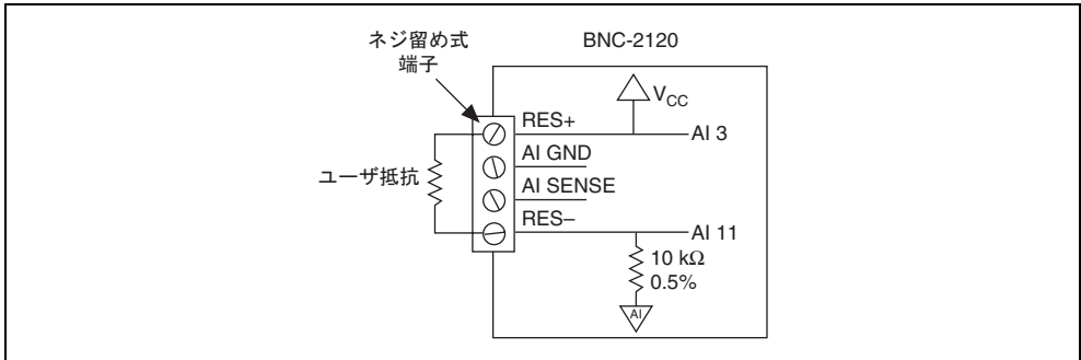
図 4 BNC-2120 で抵抗を測定する
