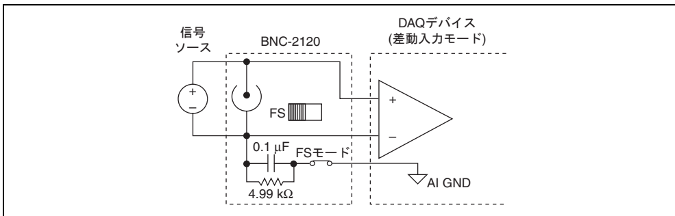
図 2 浮動型信号ソースを測定する
