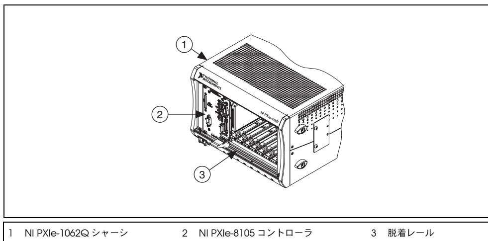
図 2 PXI Express シャーシに取り付けられた NI PXIe-8105 コントローラ
