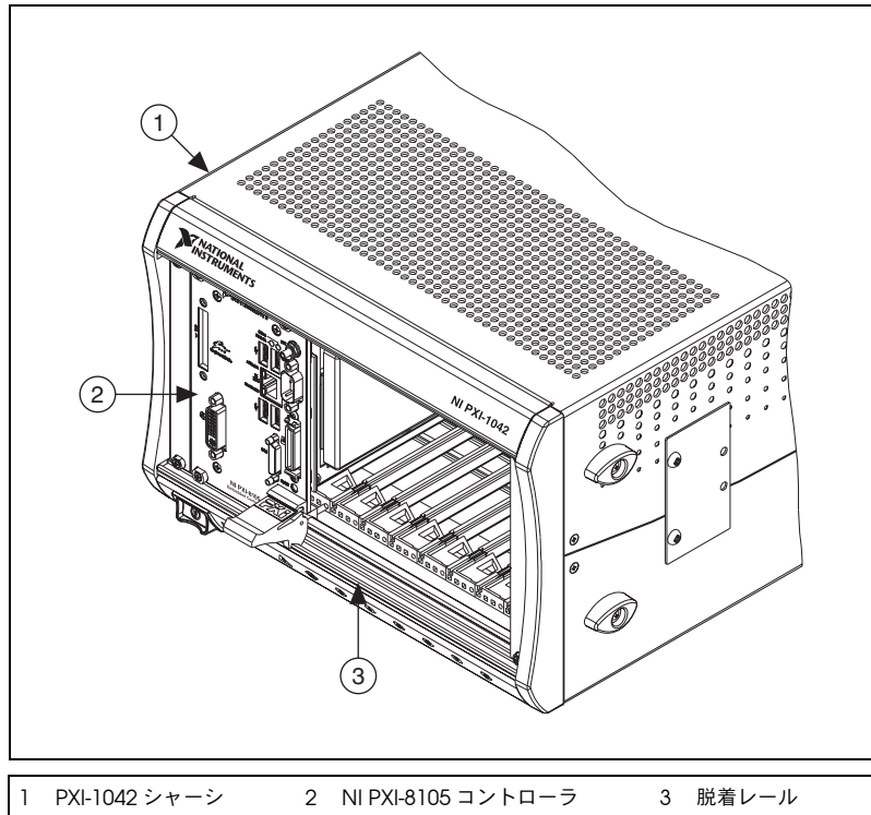
図 2-2 PXI シャーシに取り付けた NI PXI-8105 コントローラ
