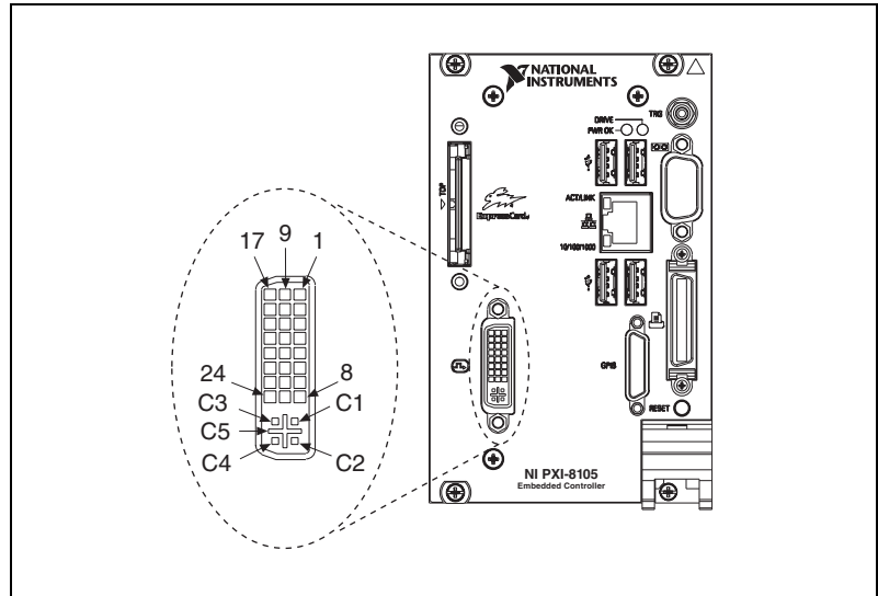
図 3-2 DVI-I コネクタの位置およびピン配列
