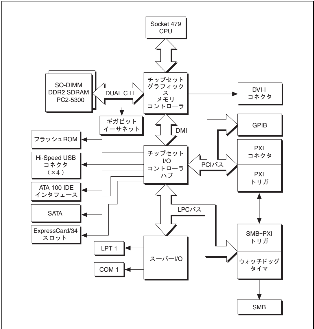
図 1-1 NI PXI-8105 ブロック図
