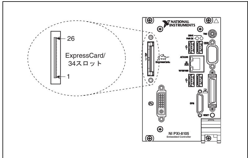
図 3-9 ExpressCard/34 スロットの位置とピン配列
