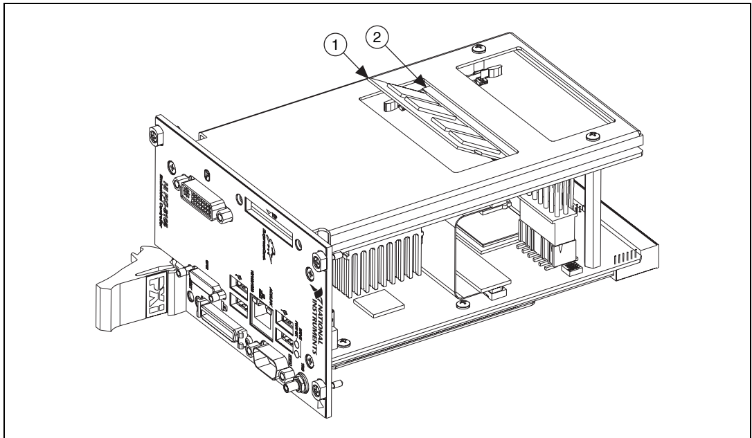
図 2-5 NI PXI-8105 コントローラに DDR2 SO-DIMM を取り付ける
