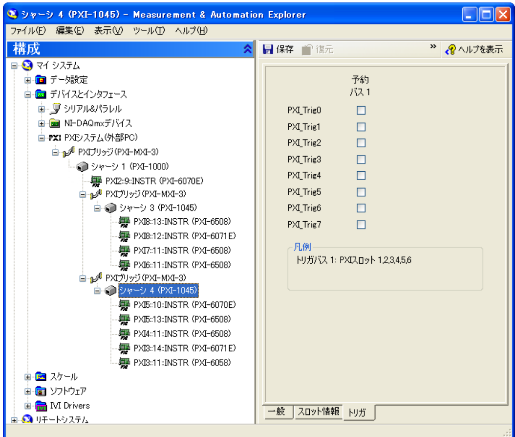
図 2-4 MAX でのマルチシャーシ構成
