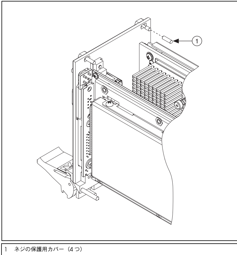
図 2-1 ネジの保護用カバーを外す
