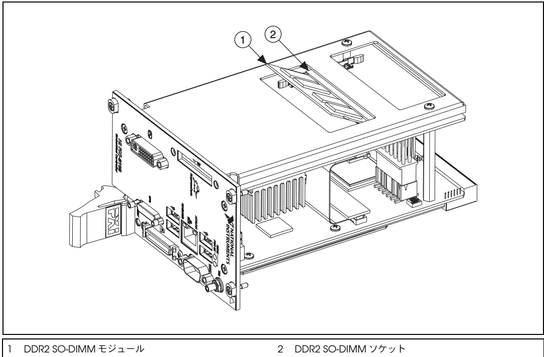
図 4-2 NI PXI-8105 コントローラに DDR2 SO-DIMM を取り付ける
