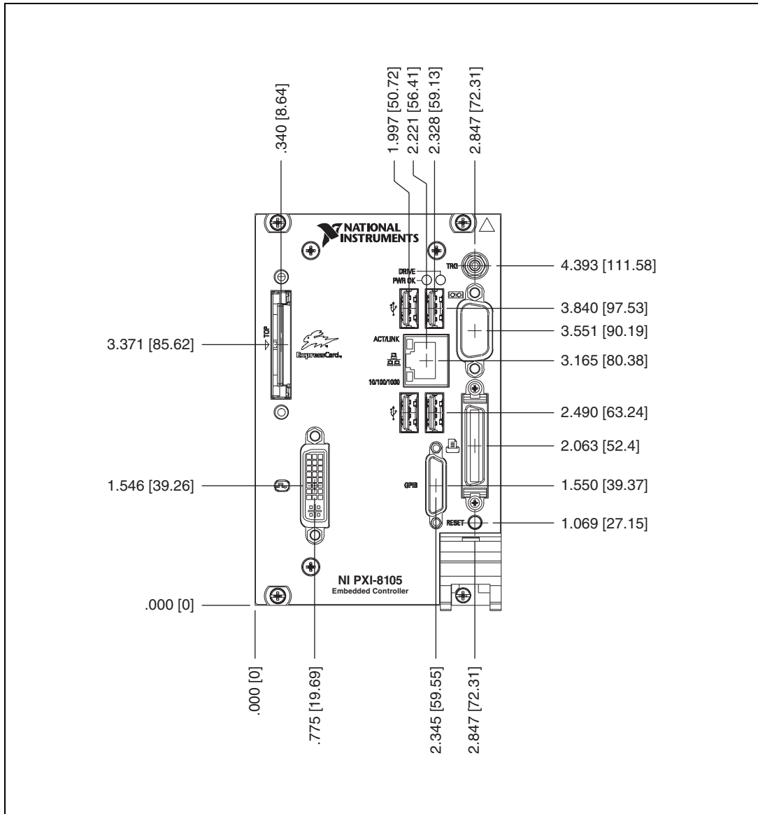
図 3-1 NI PXI-8105 フロントパネルの配置および寸法
