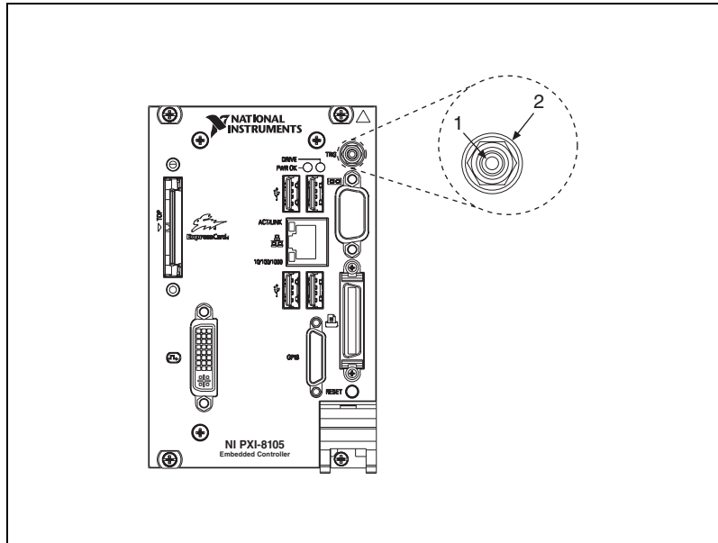
図 3-7 TRG コネクタの位置およびピン配列
